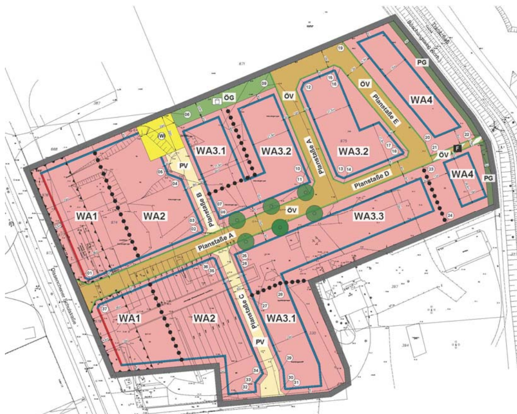
Planzeichnung
