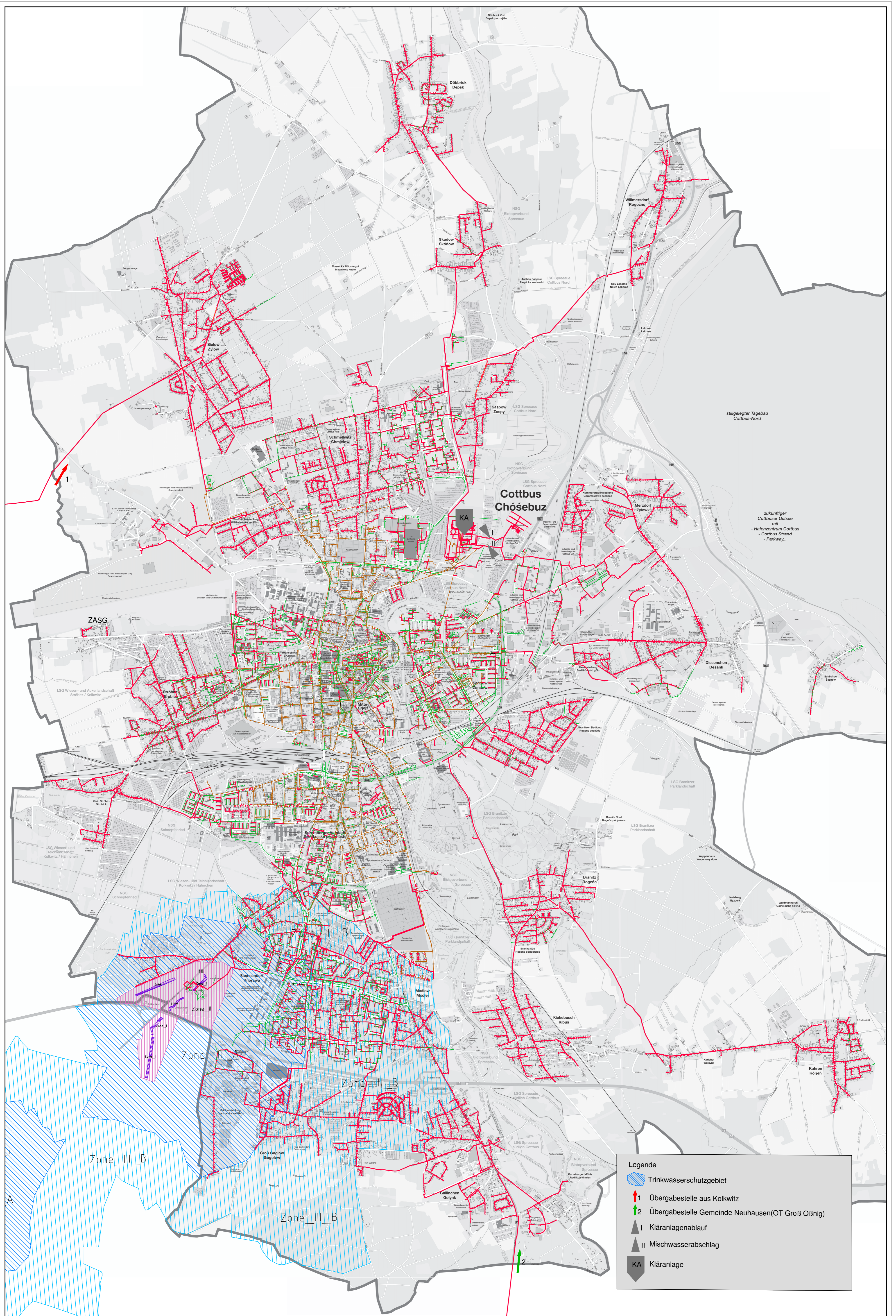
Übersichtsplan Abwasserentsorgung Kanalnetz Stadt Cottbus
